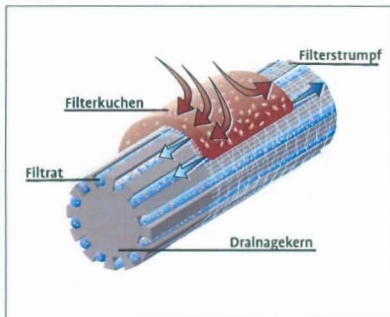
Querschnitt Drainageelement
