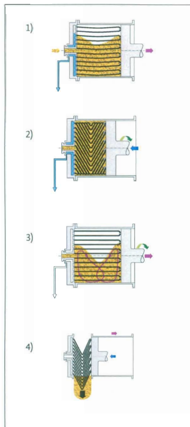
Funktionsprinzip Presse
