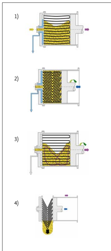
Funktionsprinzip Presse
